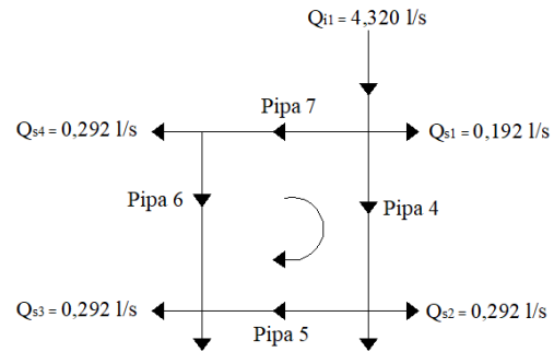
Gambar 3. Pemodelan Loop 1
