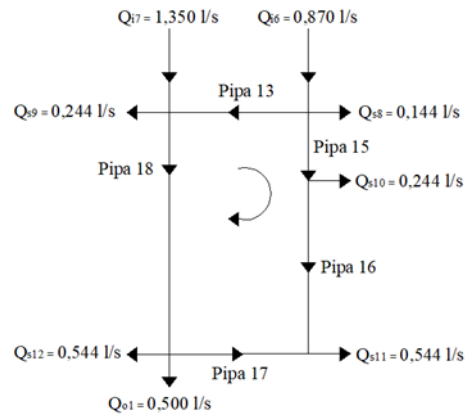
Gambar 6. Pemodelan Loop 4
