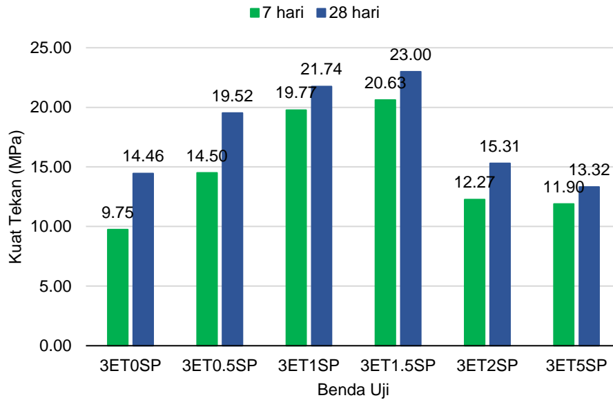
Gambar 2. Kuat Tekan Beton Pada Umur 7 hari dan 28 hari
