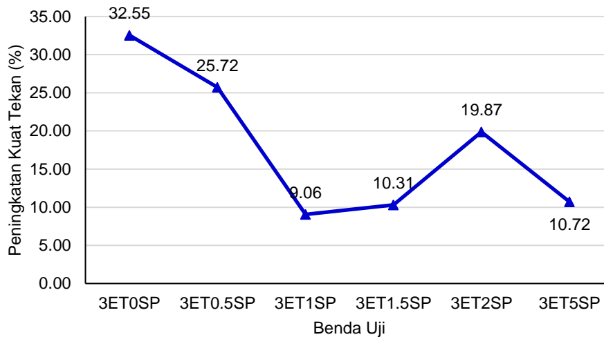
Gambar 3. Peningkatan Kuat Tekan Beton dari Umur 7 hari ke Umur 28 hari
